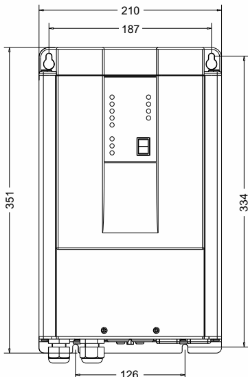
Vooraanzicht
